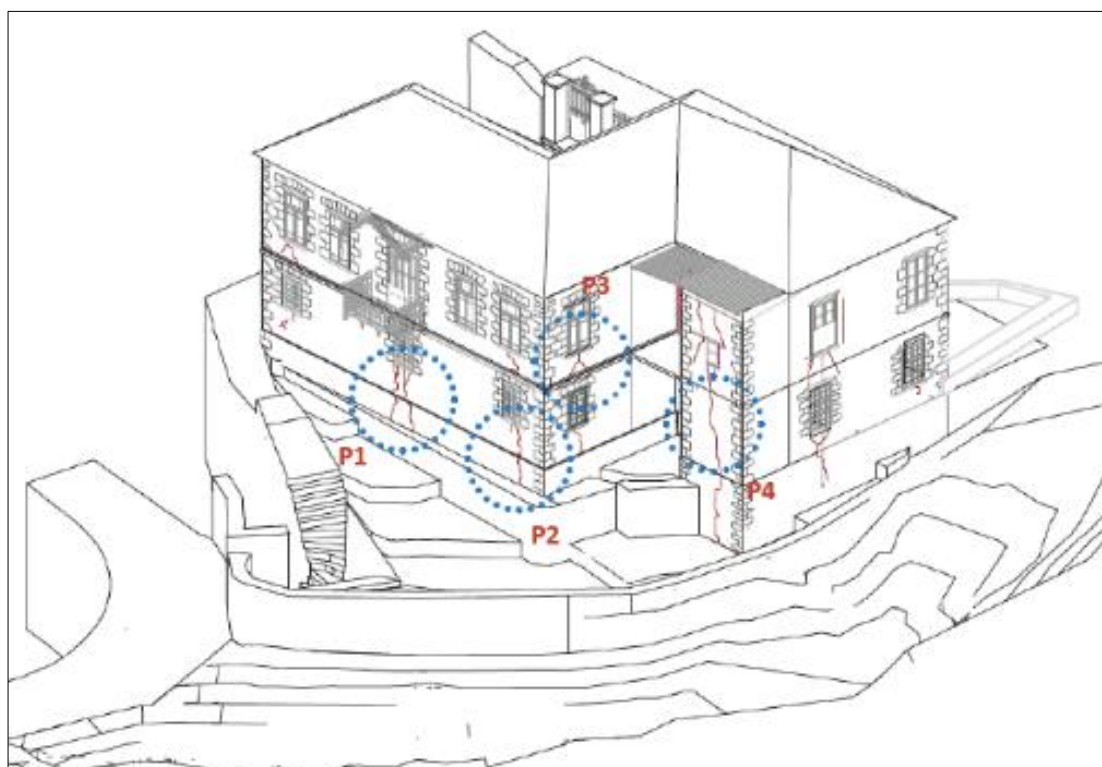
Εικόνα 3-56. Ρωγμές λόγω σεισμού κοντά στη γωνία των κτιρίων (Οικία Νικοπούλου, Οικία «του Δασκάλου», Οικία Καραγεώργου). Πηγή: Ερευνητική ομάδα ΕΜΠ, 2023. Σχέδια: Α. Βιέννα, Α. Ζαχαράκη, Ζ. Κονδύλη, Ν. Σάκκα, Β. Λασπιά, Ο. Σπυριδάκη, Α. Στεφανή, Δ. Χρήστου, μεταπτυχιακές φοιτήτριες ΔΠΜΣ «Προστασία Μνημείων» ΕΜΠ.
