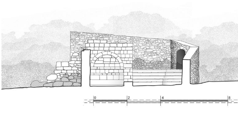
Εικόνα 5-24. Δυτική όψη της κρήνης. Κατασκευάστηκε σύμφωνα με την κτητορική επιγραφή “ΔΑΠΑΝΑΙΣ Θεοφάνους Νικόπουλου 1915”. Σχέδιο: Αποστόλης Καρκάσης, προπτυχιακός φοιτητής της Σχολής Αρχιτεκτόνων Μηχ. ΕΜΠ, Ερευνητική ομάδα ΕΜΠ, 2023.
