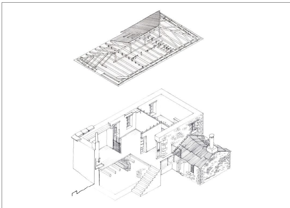
Εικόνα 3-25. Οικία «του Δασκάλου». Αξονομετρική τομή και όψεις. Πηγή: Γουγούλα Κωνσταντίνα, Καλυφόμεματος Παύλος, Ροβήλος Παναγιώτης, Ροζανή Γεωργία (Αρχιτέκτονες Μηχ.) Το σπίτι του δασκάλου στην παλαιά Βίνιανη. ΔΠΜΣ «Προστασία Μνημείων» ΕΜΠ (Μεταπτυχιακή Εργασία), Ιούλιος 2023.
