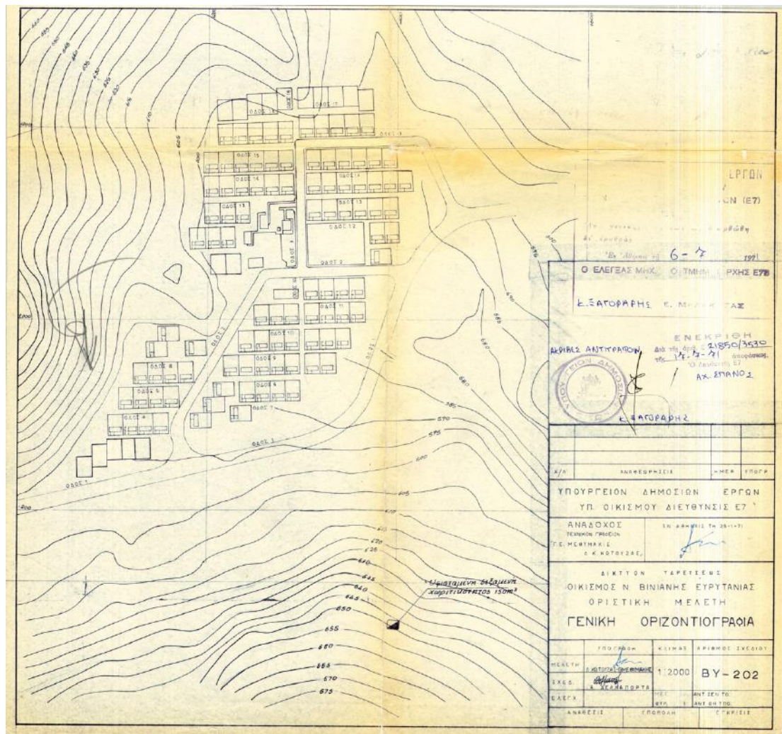
Εικόνα 5-6. Οικισμός Νέας Βίνιανης, Γενική Οριζοντιογραφία. Υπουργείον Δημοσίων Έργων, Υπ. Οικισμού, Διεύθυνσις Ε7. Πηγή: Αρχείο Σεισμοπλήκτων της Διεύθυνσης Τεχνικών Έργων της Περιφέρειας Στερεάς Ελλάδας.
