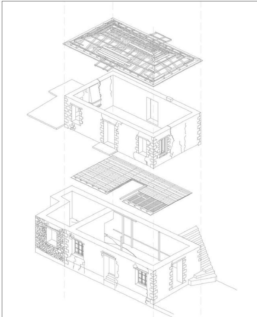
Εικόνα 3-21. Οικία Αλατάρη και Καφέ-Παντοπωλείο «Ελβετία». Αξονομετρική τομή και όψεις. Πηγή: Καραγιαννακίδου Κατερίνα, (Αρχιτέκτων Μηχ.), Κρεκούκια Νικολαΐα, (Αρχαιολόγος), Μέρου Μαρίνα, (Αρχιτέκτων Μηχ.), Κτήριο παλιού καφενείου, Βίνιανη Ευρυτανίας. ΔΠΜΣ «Προστασία Μνημείων» ΕΜΠ (Μεταπτυχιακή Εργασία), Ιούλιος 2023
