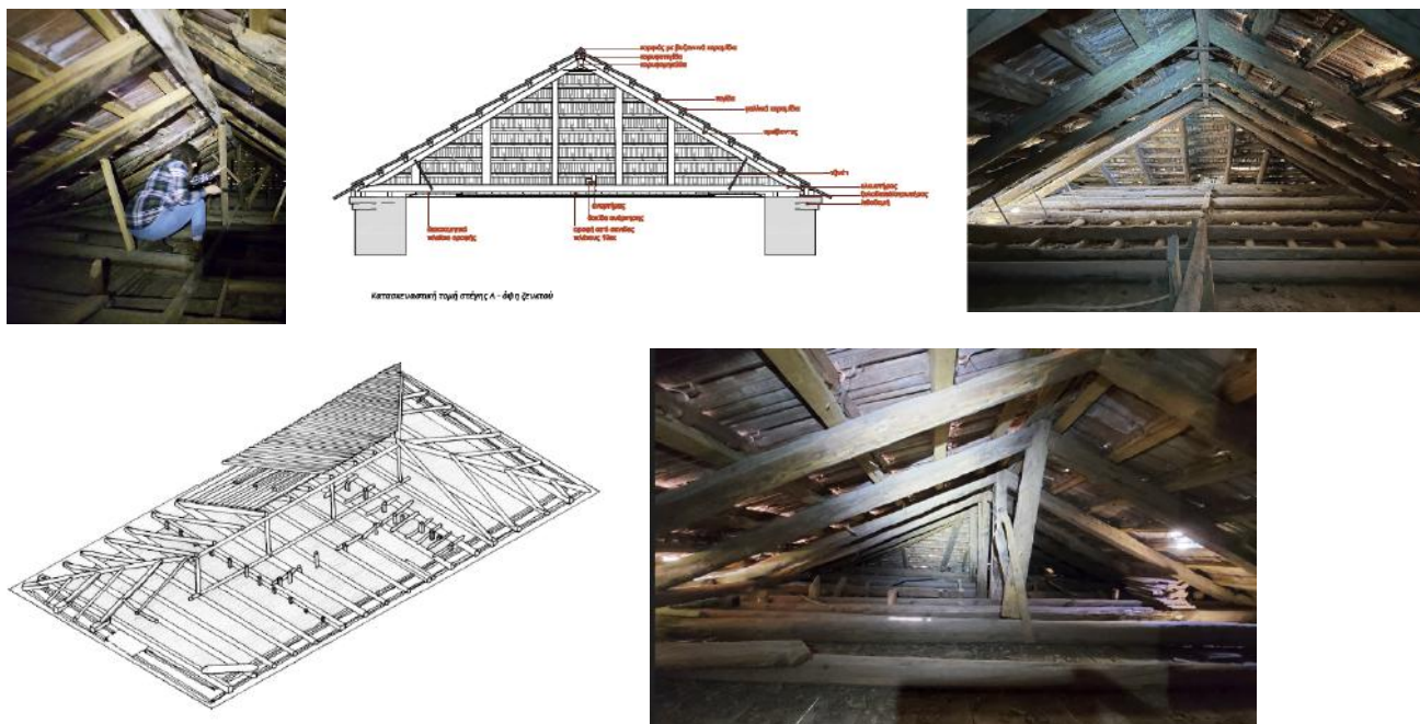
Εικόνα 3-40. Στέγες κτιρίων της Βίνιανης. Πηγή: Ερευνητική ομάδα ΕΜΠ, 2023. Σχέδια: Α. Βιέννα, Α. Ζαχαράκη, Ζ. Κονδύλη, Ν. Σάκκα, Β. Λασπιά, Ο. Σπυριδάκη, Α. Στεφανή, Δ. Χρήστου, Κ. Γουγούλα, Π. Καλυφόμεματος, Π. Ροβήλος, Γ. Ροζανή, μεταπτυχιακοί φοιτητές/τριες ΔΠΜΣ «Προστασία Μνημείων» ΕΜΠ.
