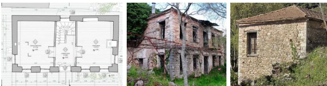
Εικόνα 3-35. Οικία Νικόπουλου: α) κάτοψη ορόφου, β) άποψη από ΝΔ και γ) άποψη από Α. Πηγή: Ερευνητική ομάδα ΕΜΠ, 2023. Σχέδια: Ε. Θεοδωράκογλου, Β. Μαντέλου, Ε. Φλώρου, Ν. Χούμα, μεταπτυχιακές φοιτήτριες ΔΠΜΣ «Προστασία Μνημείων» ΕΜΠ.
