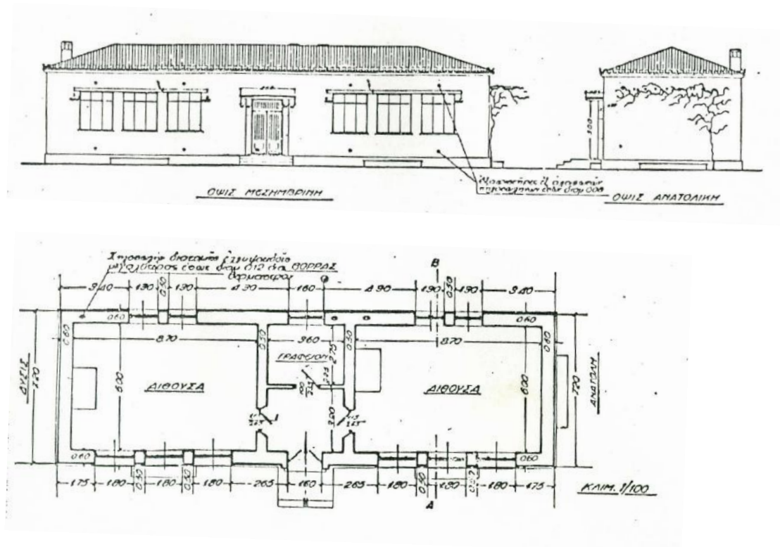
Εικόνα 3-19. Τα τυπολογικά σχέδια (κάτοψη, μεσημβρινή και ανατολική όψη) του Υπουργείου Παιδείας για τα διτάξια ορεινά σχολεία. Η τυπολογία αυτή εφαρμόστηκε στο σχολείο της Βίνιανης. Τα σχέδια του κρατικού προγράμματος σχολικής στέγης του 1930 δημοσιεύθηκαν στην έκδοση του 1938 του Τεχνικού Επιμελητηρίου Ελλάδος. Πηγή: ΤΕΕ (1938). Τα νέα σχολικά κτίρια, Αθήνα.
