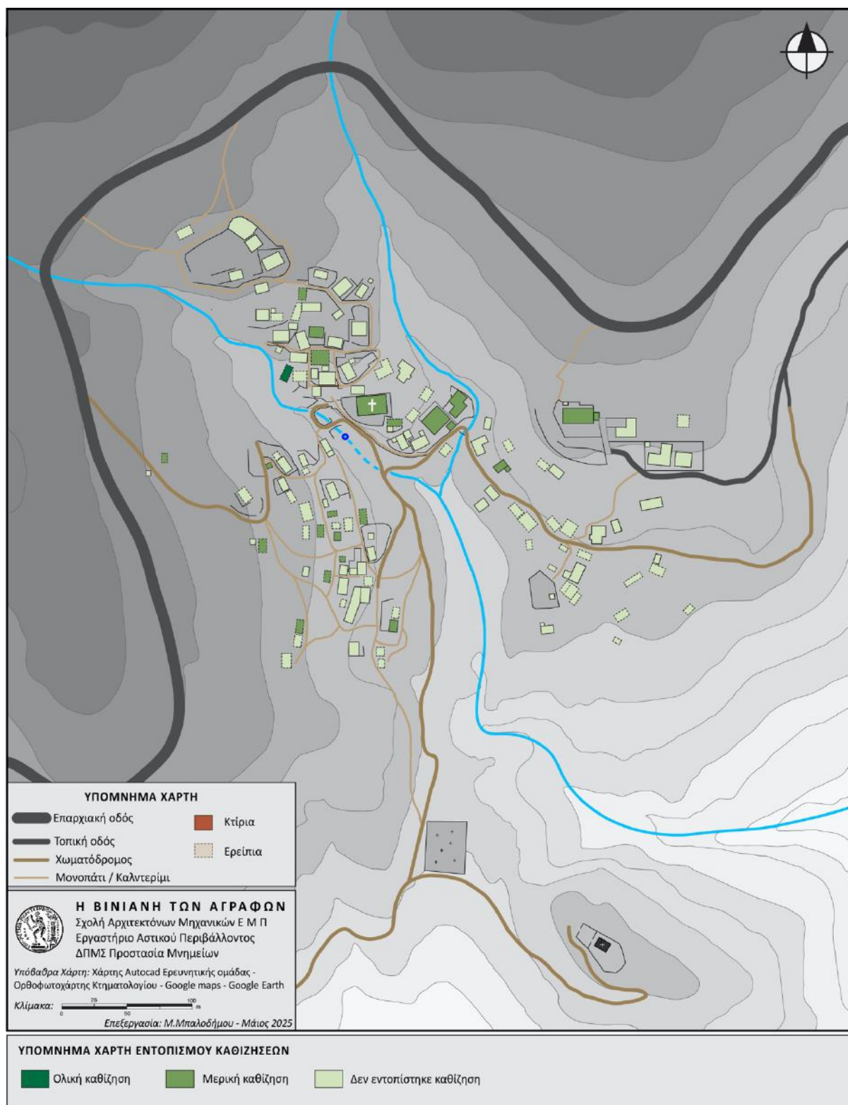
Χάρτης 5-5. Κτίρια με πρόβλημα καθίζησης στη Βίνιανη. Επεξεργασία: Ερευνητική ομάδα ΕΜΠ, 2023. Γεωγραφικό Σύστημα Πληροφοριών: Αργυρή Βιέννα, Βασιλική Λασιπιά, Αγρ. Τοπογράφοι Μηχανικοί, μεταπτυχιακές φοιτήτριες ΔΠΜΣ «Προστασία Μνημείων». Επιτόπιες καταγραφές: Χάρις Βράκα, Αποστόλης Καρκάσης, Αθηνά Κούρκουλου, Χάρης Λυσικάτος, Κάλλη Μπούρχα, Ζωή Ριζάκη, Νότα Στράγκα, Μαρία Χριστοδούλου, προπτυχιακοί φοιτητές/τριες της Σχολής Αρχιτεκτόνων Μηχ. ΕΜΠ.
