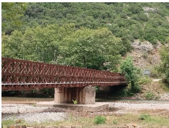
Εικόνα 3-60. Η γέφυρα τύπου Μπέιλι έχει ενισχυμένα βάθρα μπετόν αρμέ. Απαιτείται στοιχειώδης συντήρηση των μεταλλικών της στοιχείων. Πηγή: Ερευνητική ομάδα ΕΜΠ, 2023.
