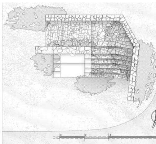
Εικόνα 5-23. Κάτοψη και φωτογραφία της κρήνης. Δίπλα της υπήρχαν τα στεγασμένα κοινοτικά πλυσταριά «καζαναριά». Κατασκευάστηκε σύμφωνα με την κτητορική επιγραφή “ΔΑΠΑΝΑΙΣ Θεοφάνους Νικόπουλου 1915”. Σχέδιο: Αποστόλης Καρκάσης, προπτυχιακός φοιτητής της Σχολής Αρχιτεκτόνων Μηχ. ΕΜΠ, Ερευνητική ομάδα ΕΜΠ, 2023.
