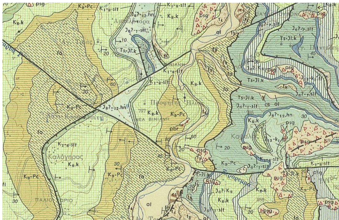
Εικόνα 4-1. Τμήμα του γεωλογικού χάρτη «Φραγκίστα», κλίμακας 1:50.000, με την περιοχή της Βίνιανης. Πηγή: Ινστιτούτο Γεωλογικών Μελετών (ΙΓΜΕ).
