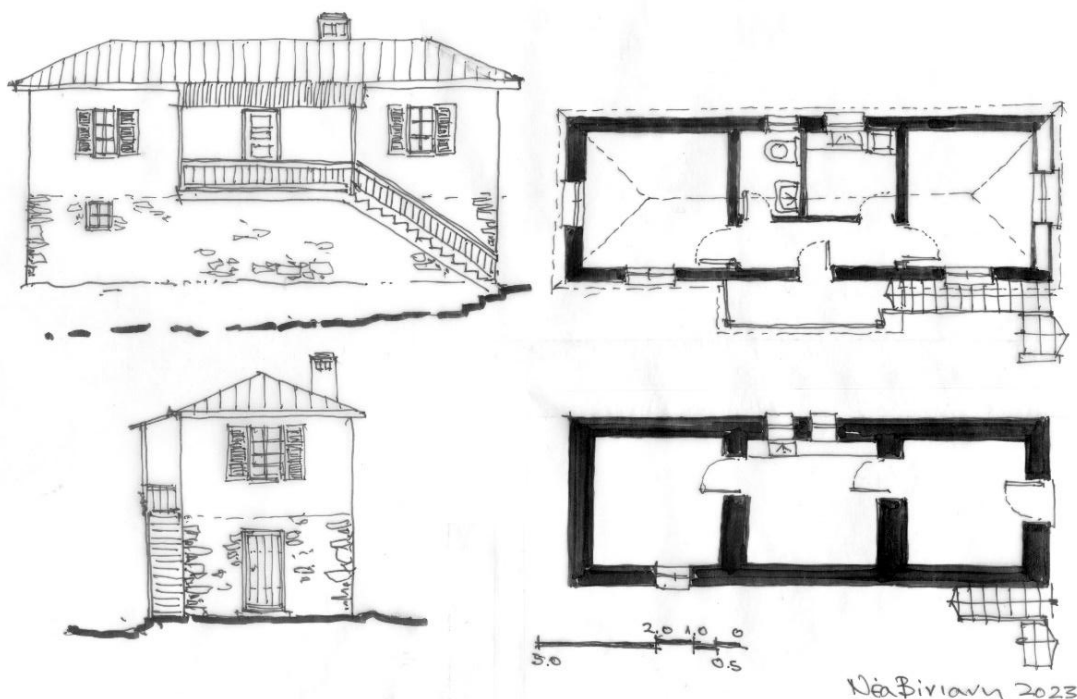
Εικόνα 5-16. Τύπος κατοικίας διώροφης με τρεις χώρους στο ισόγειο «κατώι», ένα υπνοδωμάτιο, μαγειρείο, λουτρό, διάδρομο εισόδου, στεγασμένο εξώστη και εξωτερική κλίμακα ανόδου. Κάτοψη και όψεις. Νέα Βίνιανη. Πηγή: Ερευνητική Ομάδα ΕΜΠ, Ιούνιος 2023.
